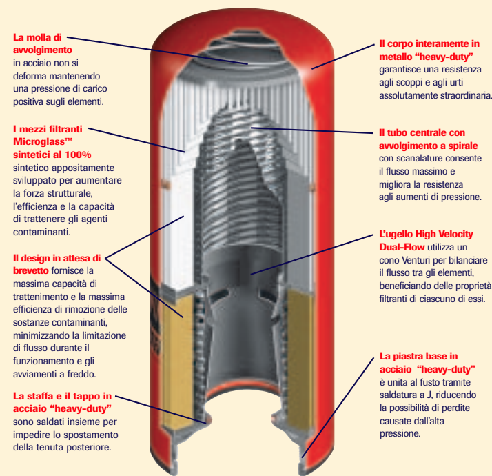
L'illustrazione raffigura i modelli BD7153 e BD7154. Il modello BD7309 utilizza una piastra base in acciaio con saldatura a doppia piega.
